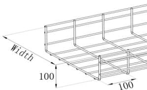
上图为标准的网格桥架300(W)剖面图
